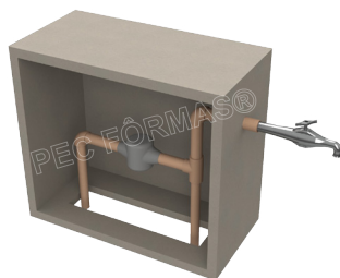
Fôrma para Abrigo de Cavalete D'água ou Gás
